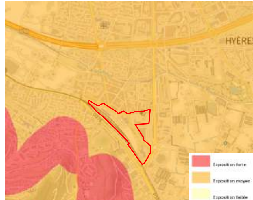
Figure 4 : Aléa Retrait-gonflement des argiles (Source : Géorisques)
